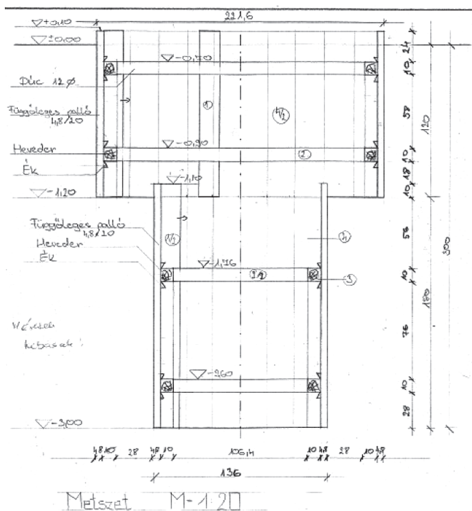
3. ábra. Munkaárok megtámasztásának metszete (készítette: Kőmives Norbert 13. osztály)
