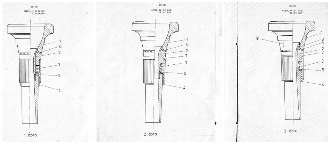
65. ábra: Rác Rudolf - rúgós fúvóka
