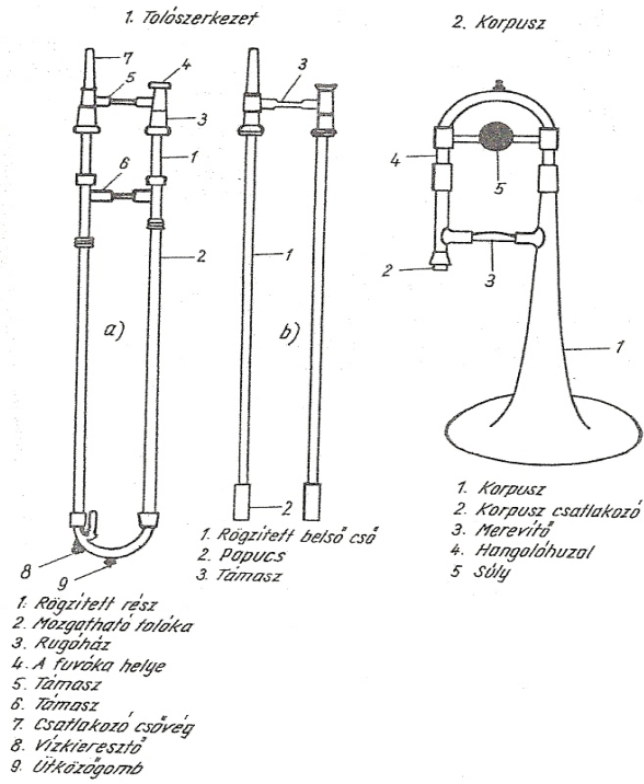
11. ábra: A harsona szerkezeti felépítése
